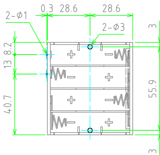
取付穴加工寸法
