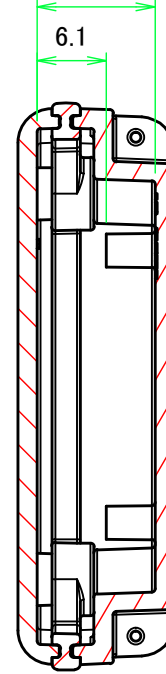
B-B ( 1.5 : 1 ) 有効寸法 / Max dim. 10.4
