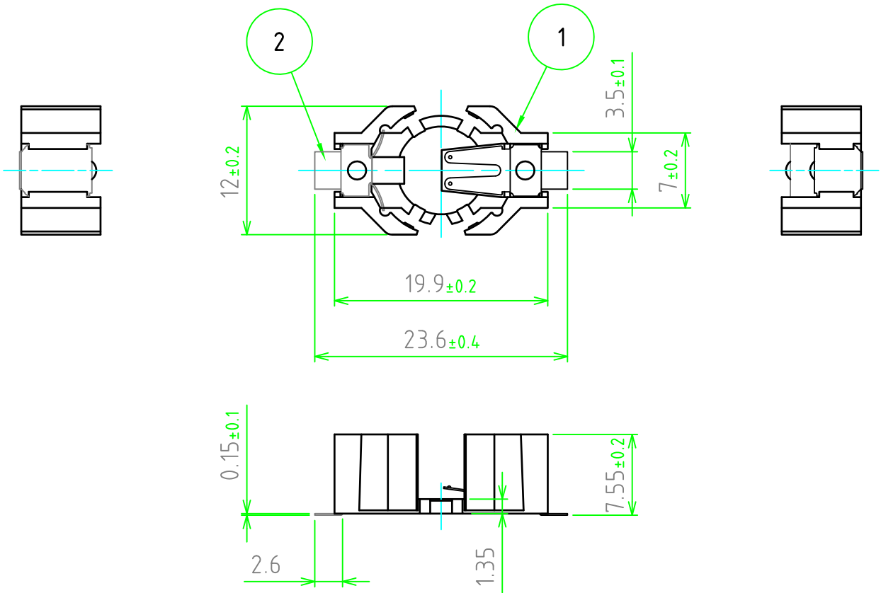
基板実装図
