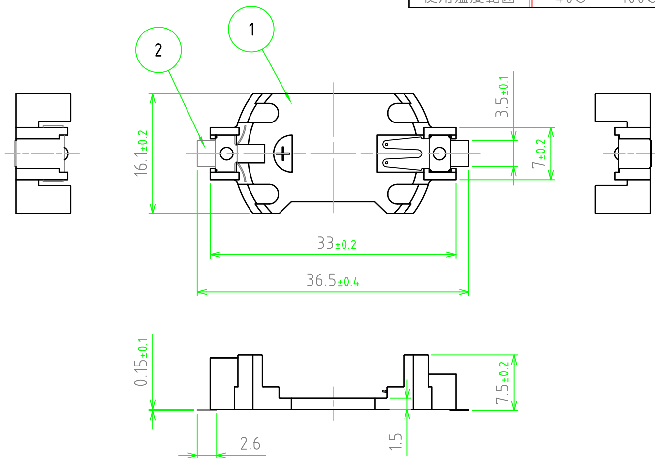
基板実装図
