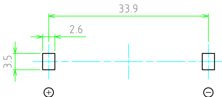
基板実装図
