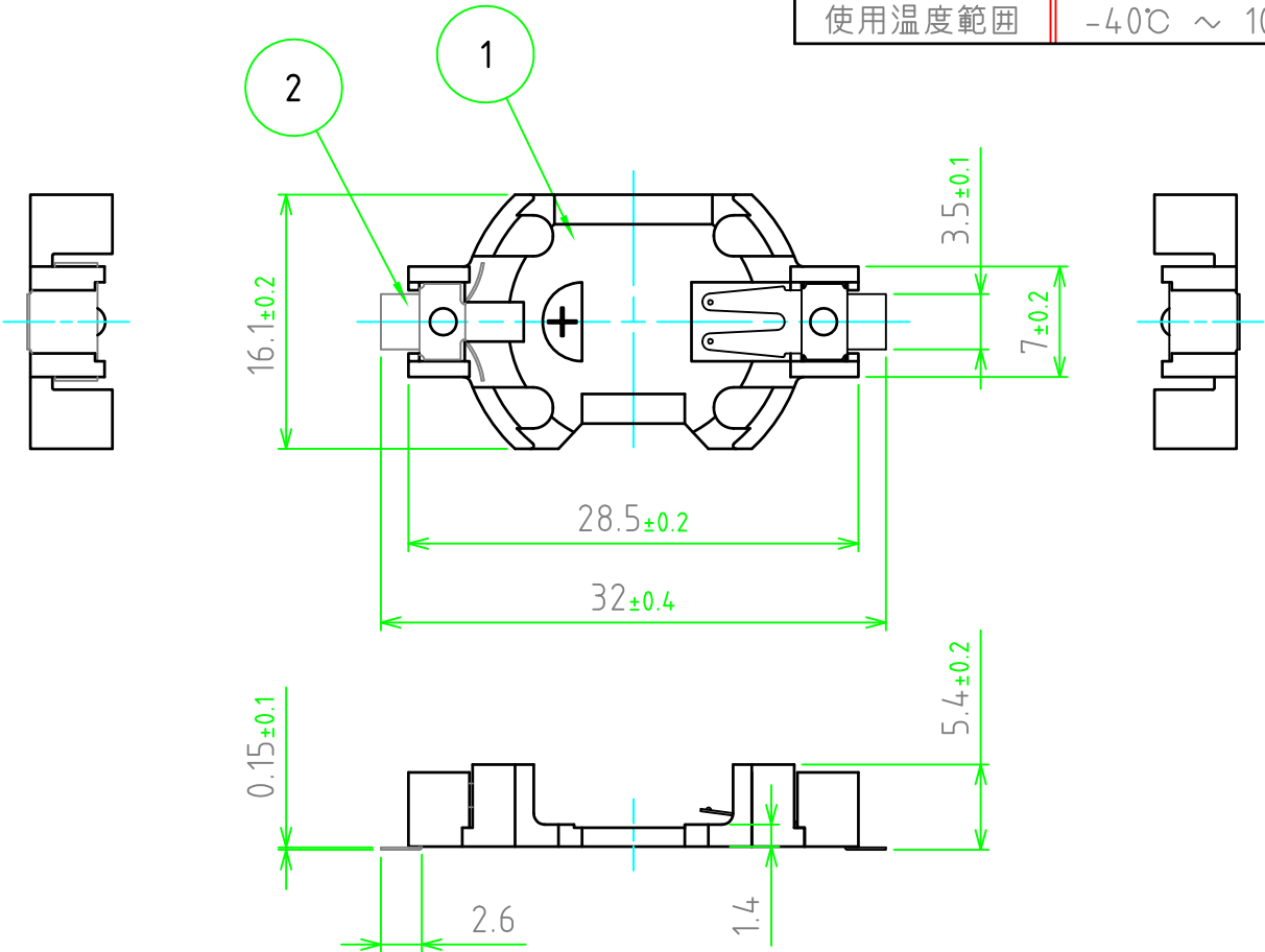
基板実装図
