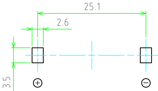
基板実装図
