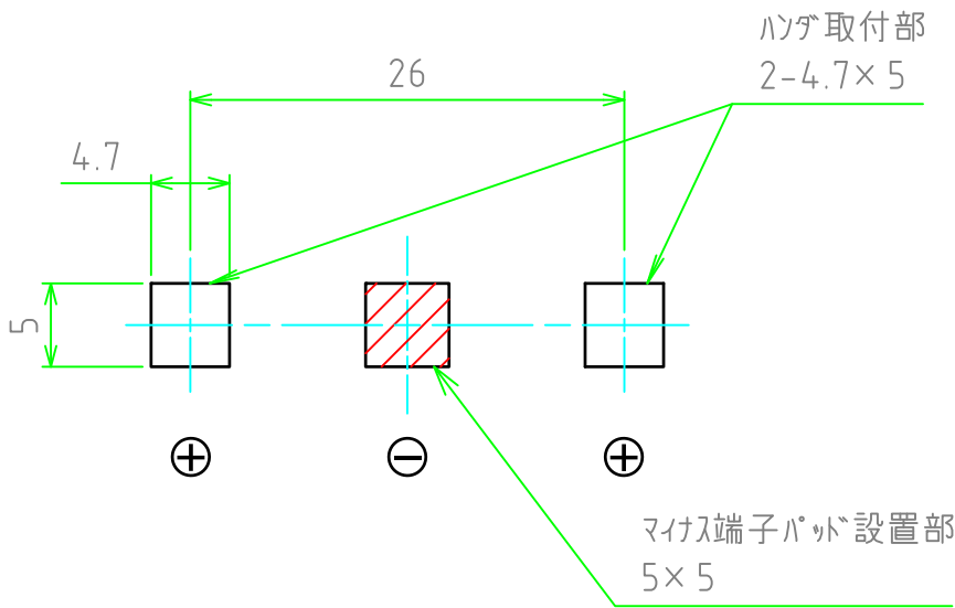
基板実装図
