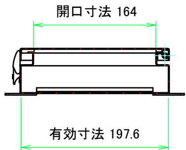
A-A (1:5)
