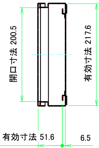
B-B ( 1 : 5 )
