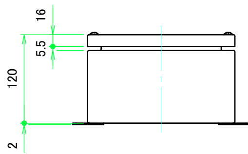
A-A (1:5)
