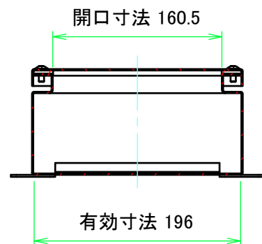
A-A (1:5)
