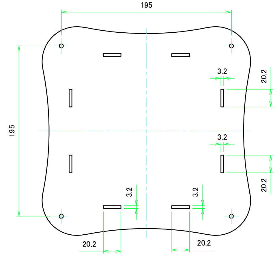
上カバー裏面 / Top cover Backside
