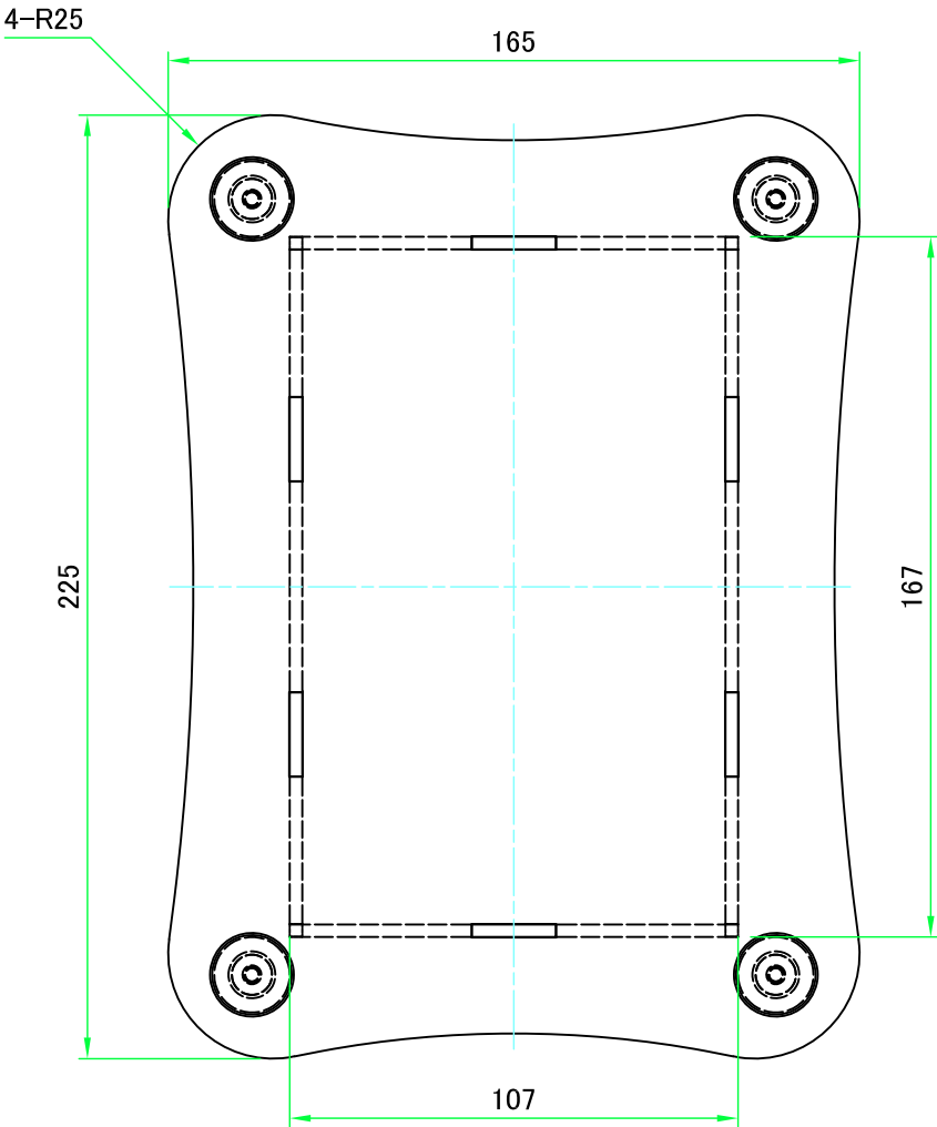
上カバー / Top cover
