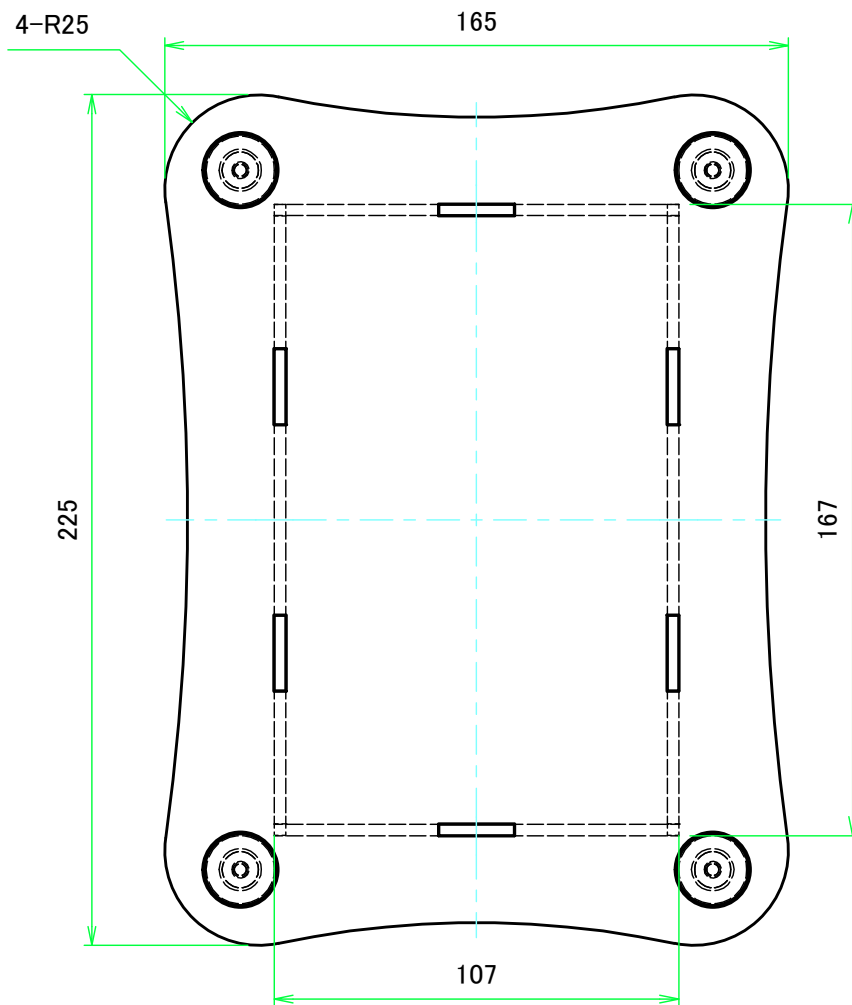
上カバー / Top cover
