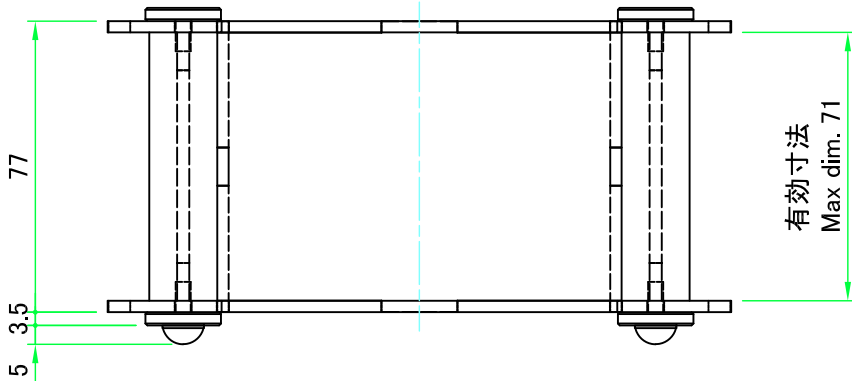
Wパネル1 / W Panel 1
