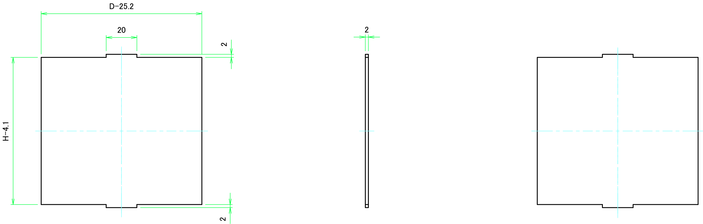
Dパネル1表面 / D Panel 1 Frontside
