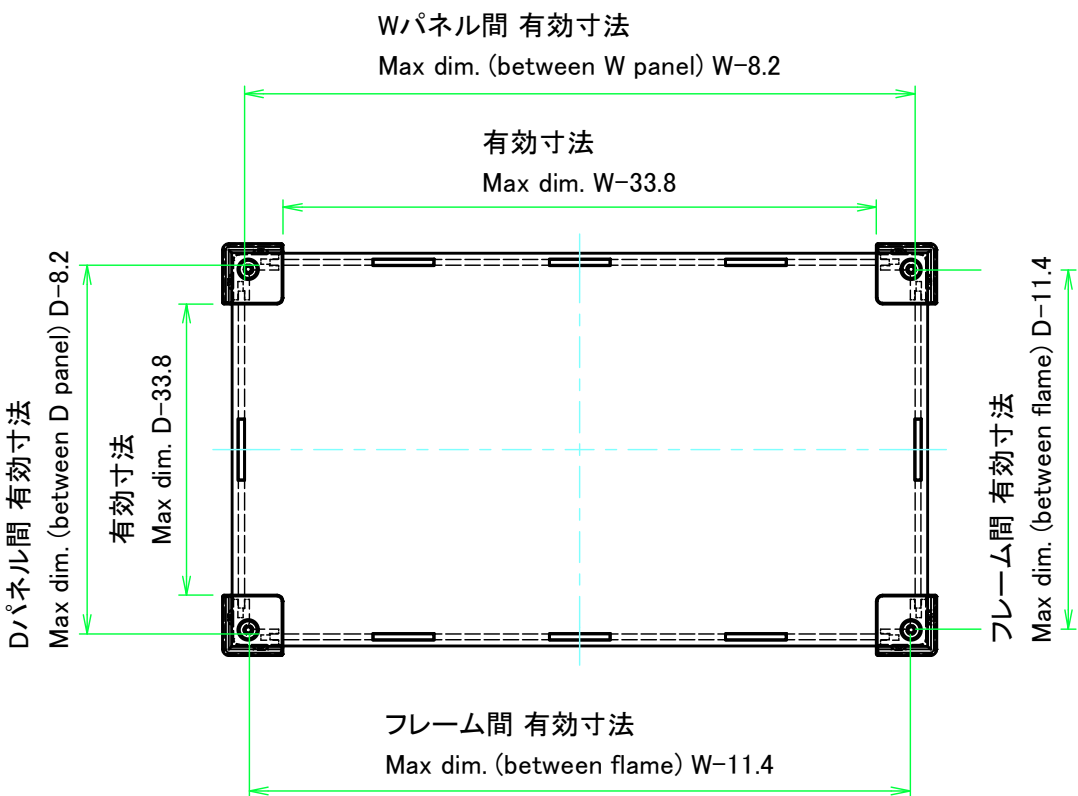
下カバー / Bottom cover
