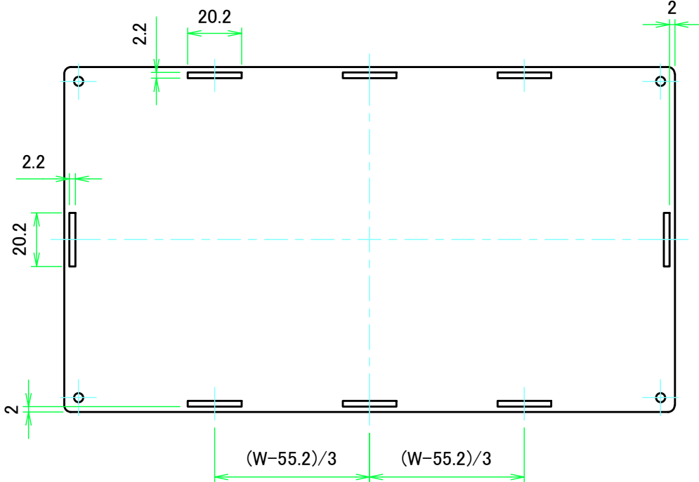
上カバー裏面 / Top cover Backside
