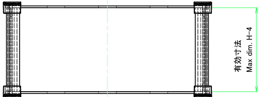
Wパネル1 / W Panel 1
