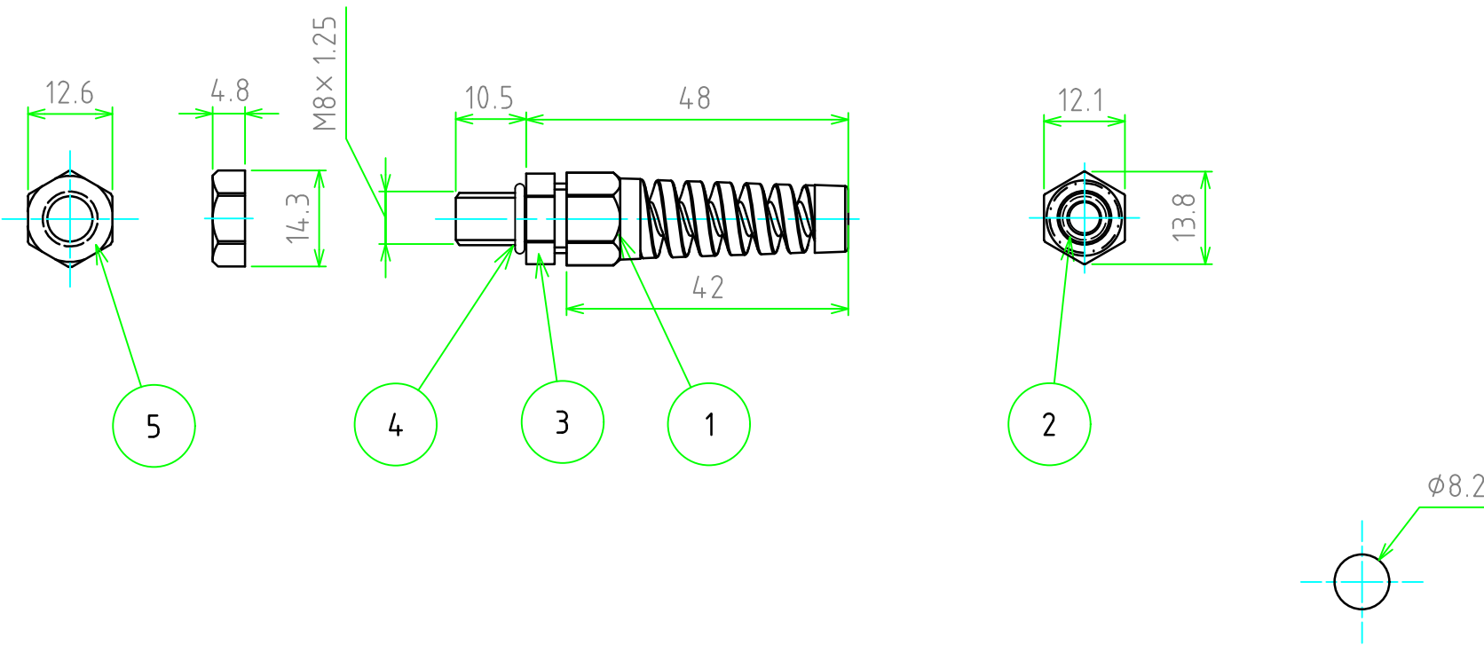
取付穴寸法 / Mounting hole dimensions
