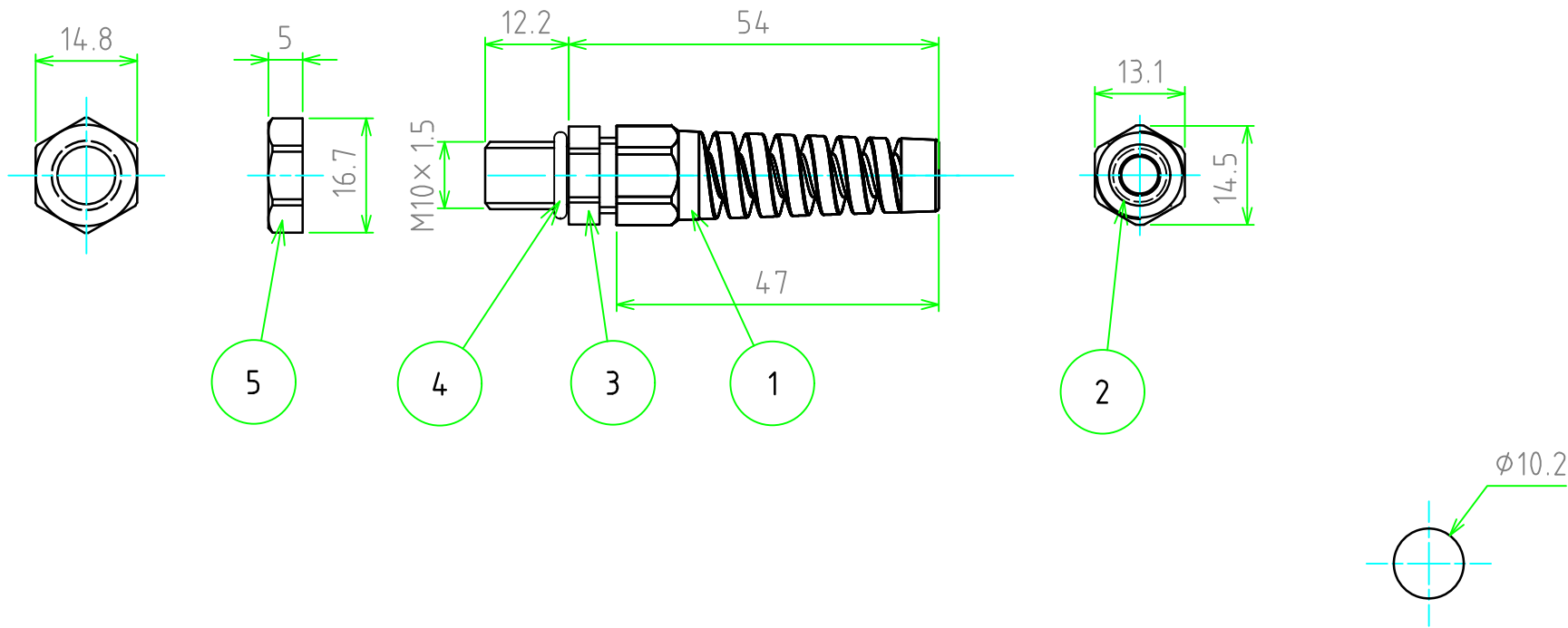
取付穴寸法 / Mounting hole dimensions
