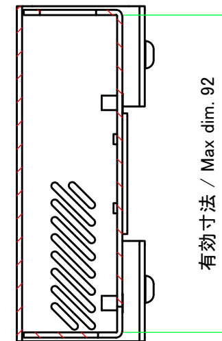
B-B ( 1 : 1.5 )
