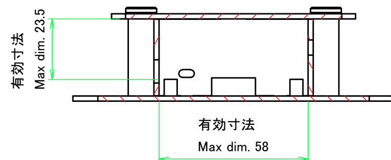
A-A ( 1 : 1.5 )
