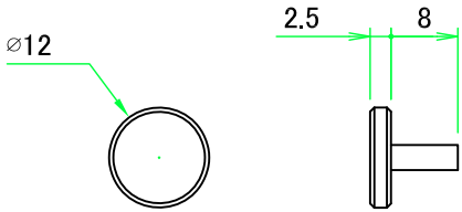
取付用ローレットビス / Knurled Thumb Screw
