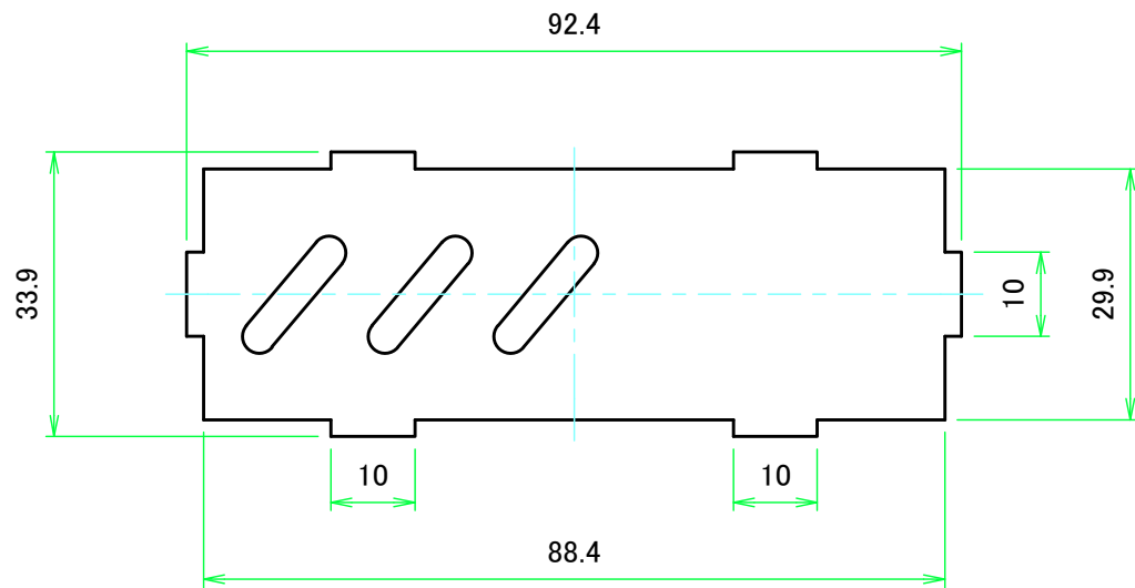
Dパネル裏面 / D Panel Backside
