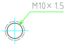
取付穴寸法 / Mounting hole dimensions
