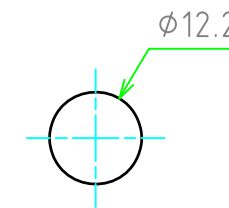
取付穴寸法 / Mounting hole dimensions
