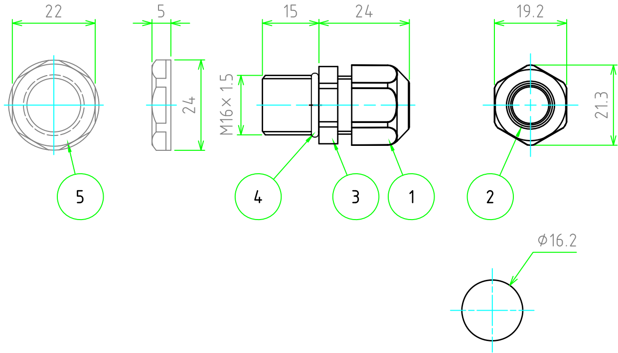
取付穴寸法 / Mounting hole dimensions
