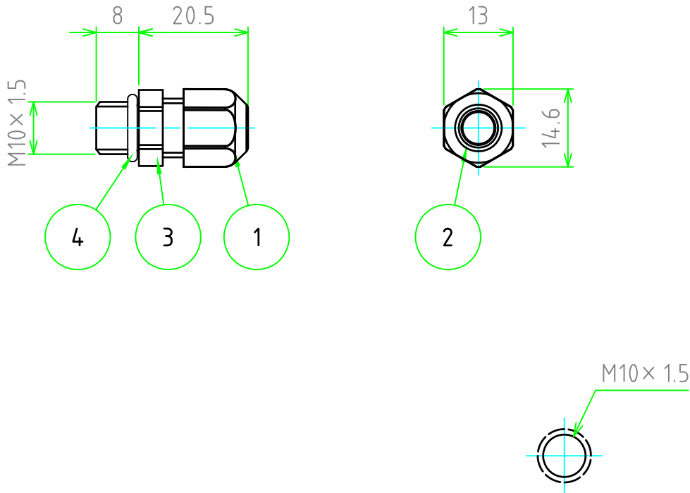
取付穴寸法 / Mounting hole dimensions
