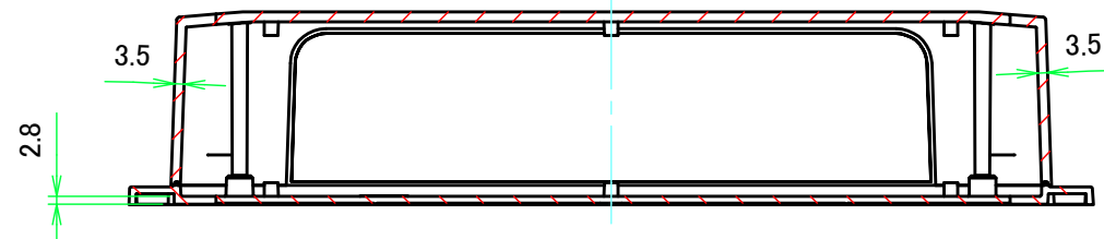
B-B ( 1 : 3 )
