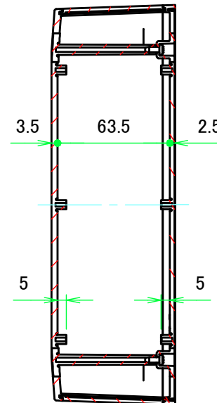
A-A ( 1 : 3 )
