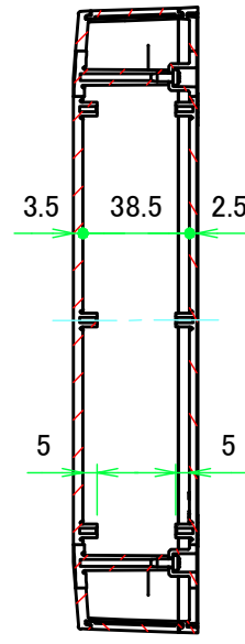
A-A (1:3)
