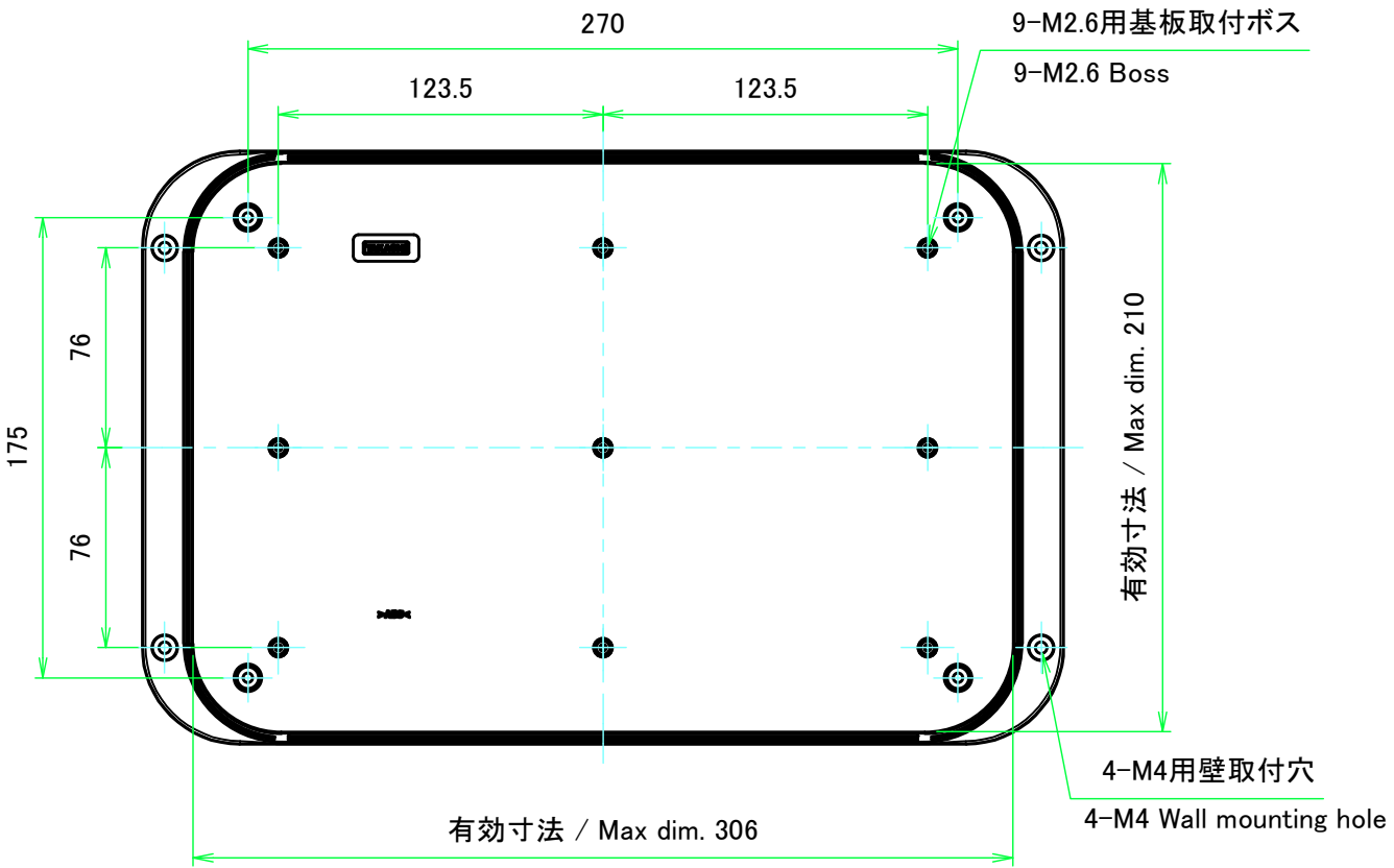
E-E ( 1 : 3 )
