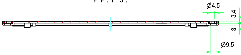
F-F ( 1 : 3 )
