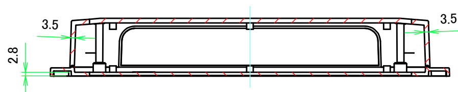
B-B ( 1 : 3 )
