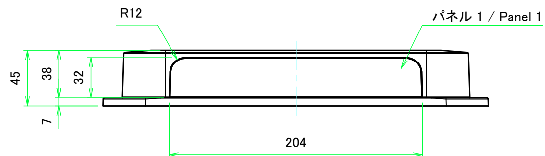
B-B ( 1 : 3 )
