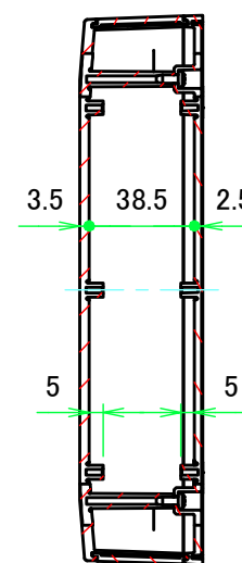
A-A ( 1 : 3 )
