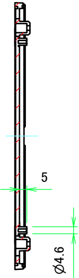
E-E ( 1 : 2.5 )
