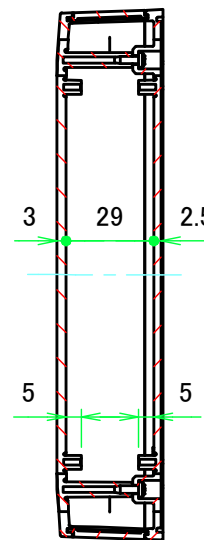
A-A ( 1 : 2.5 )
