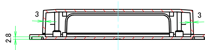
B-B ( 1 : 2.5 )
