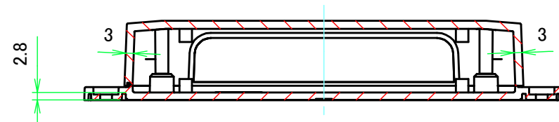
B-B ( 1 : 2 )
