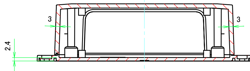
B-B ( 1 : 1.5 )
