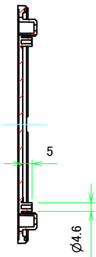
E-E ( 1 : 2 )
