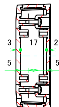
A-A ( 1 : 1.5 )
