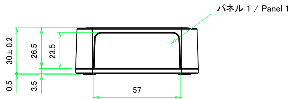
B-B ( 1 : 1.5 )
