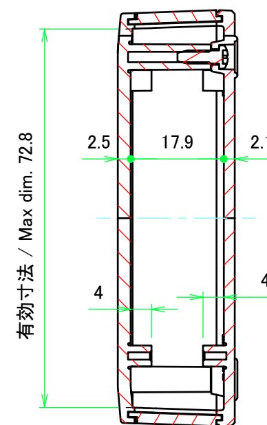
A-A (1:1)
