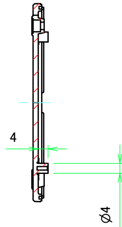
E-E ( 1 : 1.5 )
