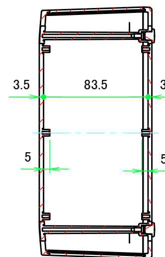
A-A (1:3)
