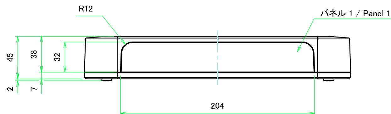
B-B ( 1 : 2.5 )
