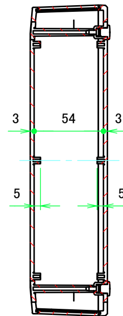
A-A ( 1 : 3 )
