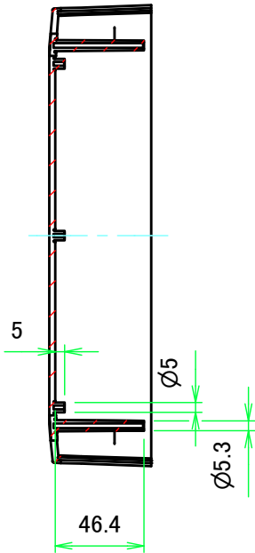
C-C ( 1 : 3.5 )
