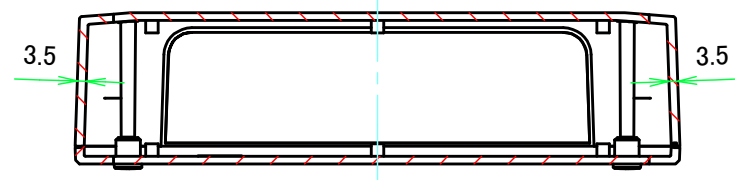
B-B ( 1 : 3 )
