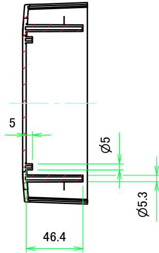
C-C ( 1 : 3 )
