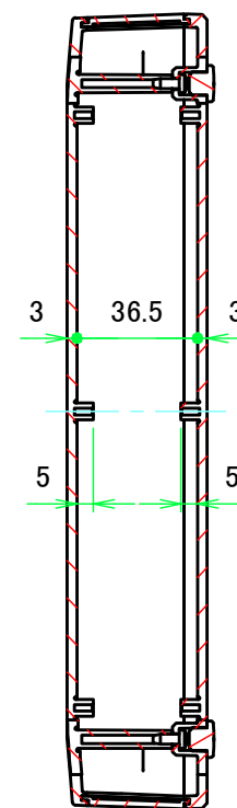
A-A ( 1 : 2.5 )
