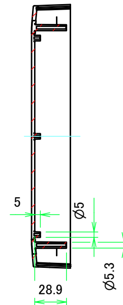
C-C ( 1 : 3.5 )
