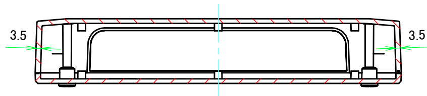
B-B ( 1 : 2.5 )
