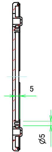
E-E ( 1 : 2.5 )
