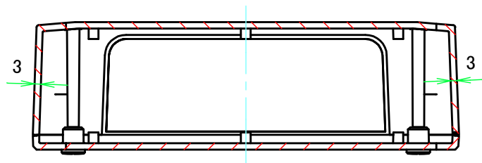
B-B ( 1 : 2.5 )
