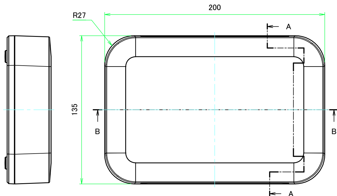
パネル 2 / Panel 2
