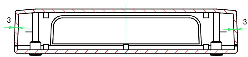
B-B ( 1 : 2 )
