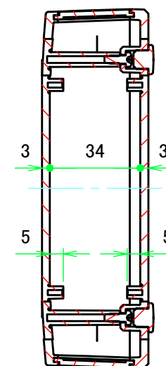
A-A ( 1 : 2 )
