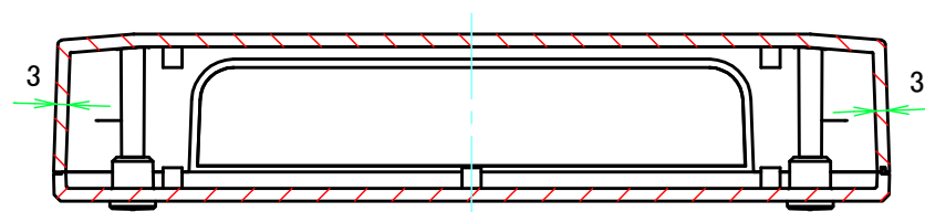
B-B ( 1 : 2 )
