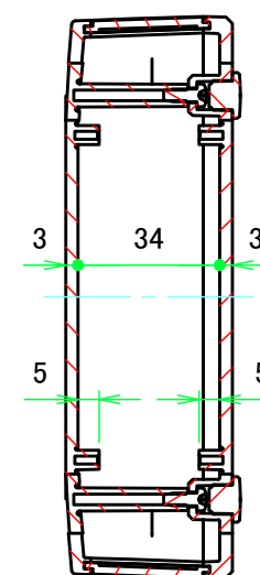
A-A ( 1 : 2 )
