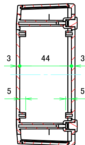
A-A ( 1 : 2 )
