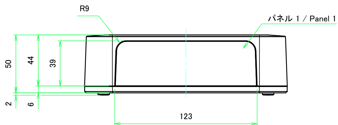
B-B ( 1 : 2 )
