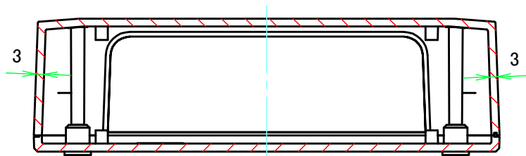
B-B ( 1 : 2 )
