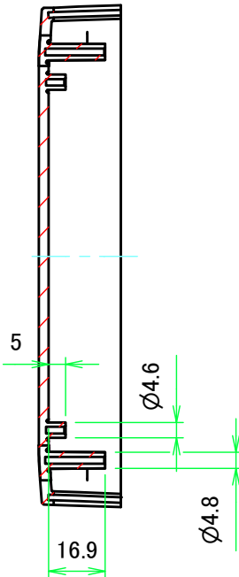
C-C ( 1 : 2 )
