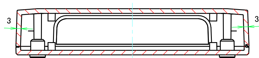
B-B ( 1 : 1.5 )
