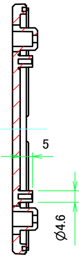
E-E ( 1 : 1.5 )
