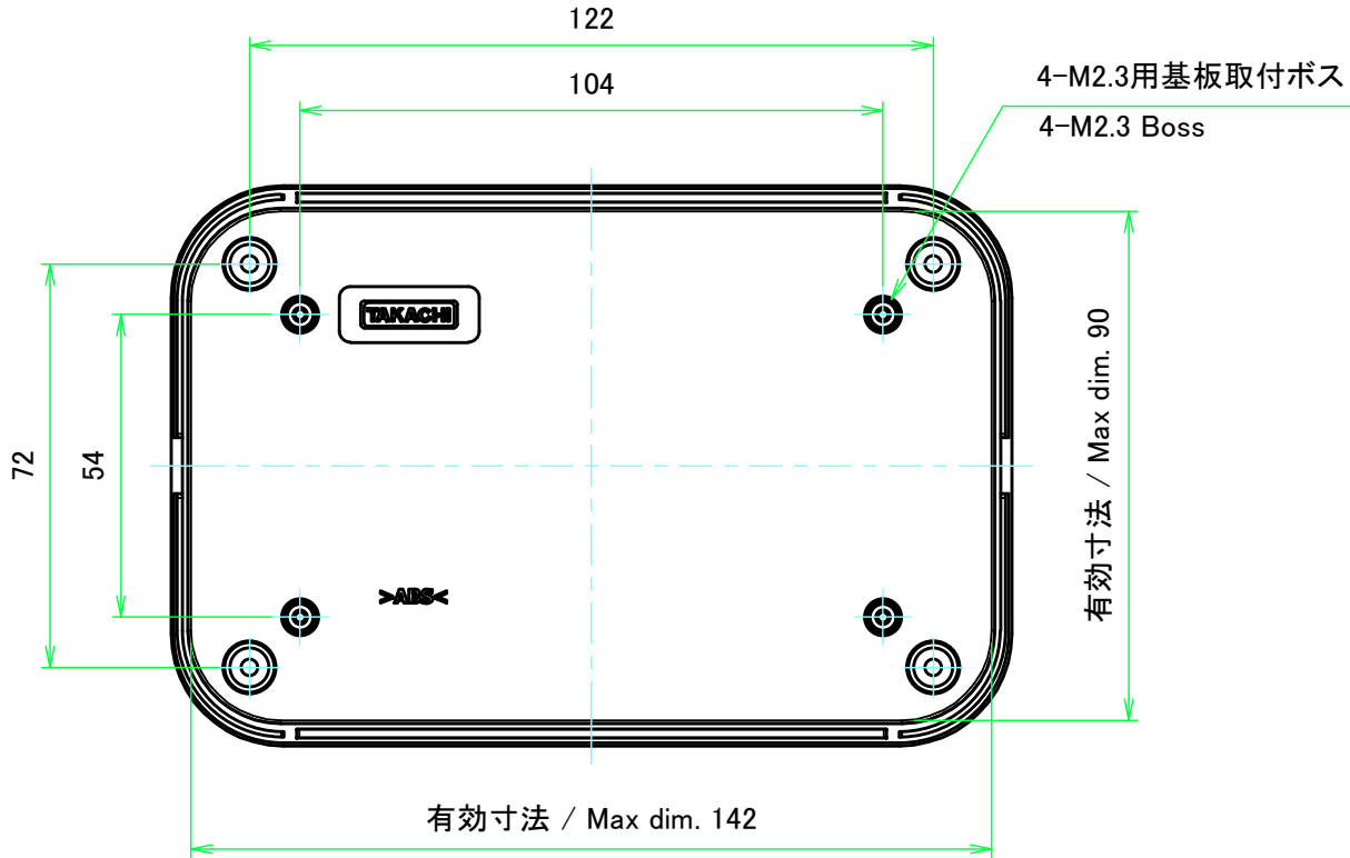
E-E ( 1 : 1.5 )
