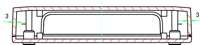
B-B ( 1 : 1.5 )
