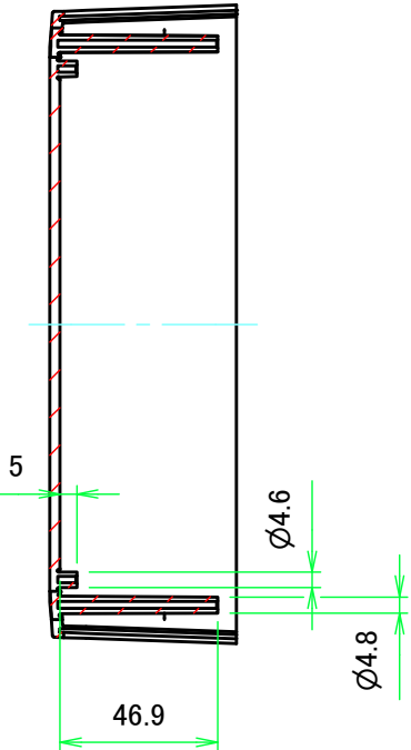
C-C ( 1 : 2.5 )
