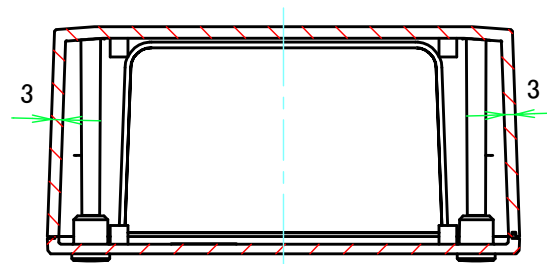
B-B ( 1 : 2 )
