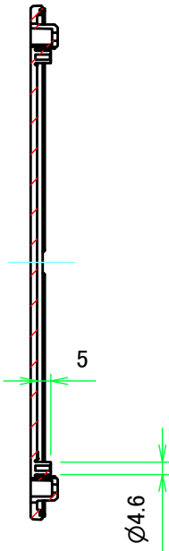
E-E ( 1 : 2.5 )
