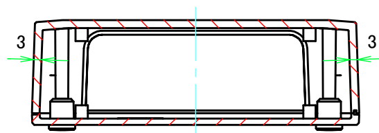
B-B ( 1 : 2 )
