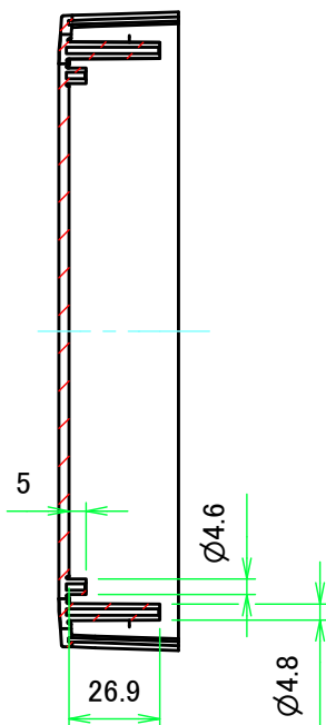
C-C ( 1 : 2.5 )
